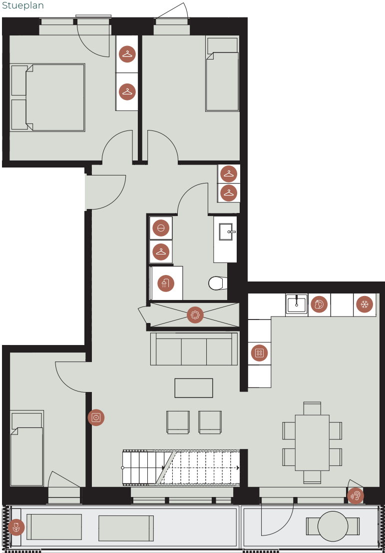
Stueplan
